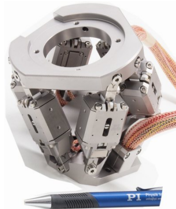
Custom miniature piezo hexapod
